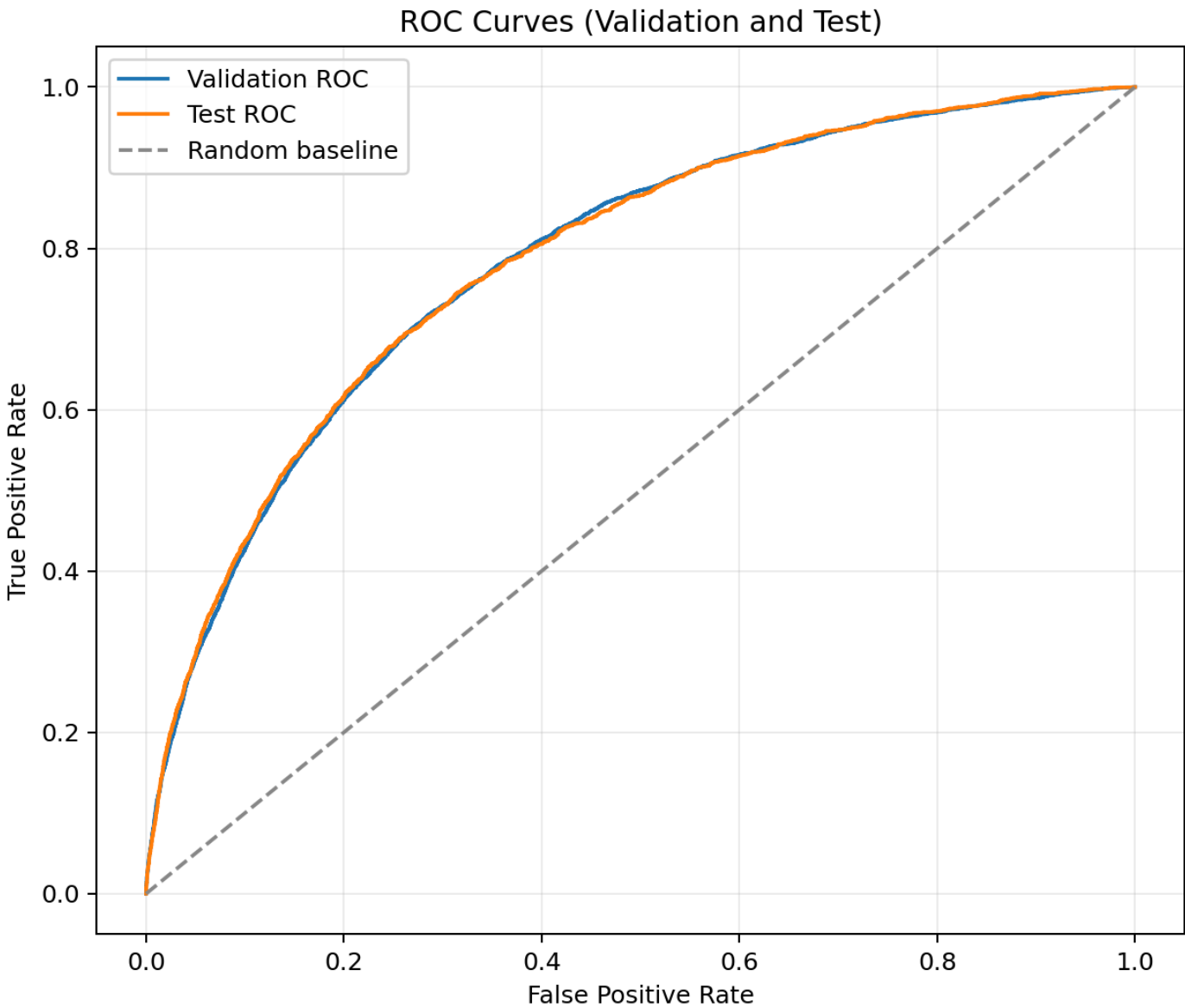
figure2_roc_curve_validation_test.png
